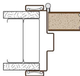
1A Jamb Hinge Side
